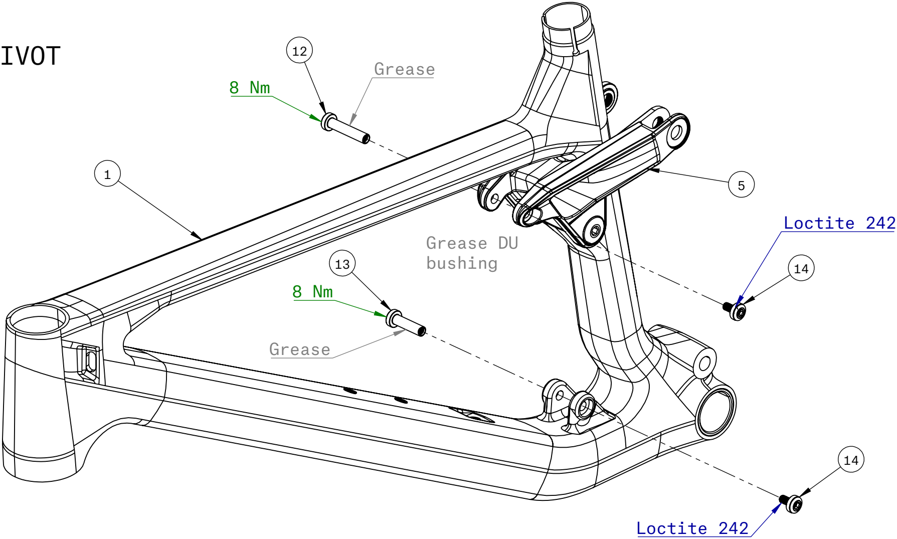
SHOCK PIVOTS
